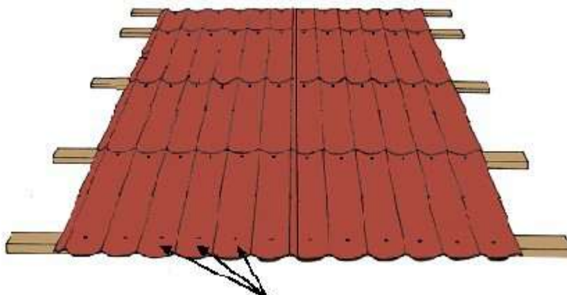
En skrue i hver bølgebund i nederste lægte.
